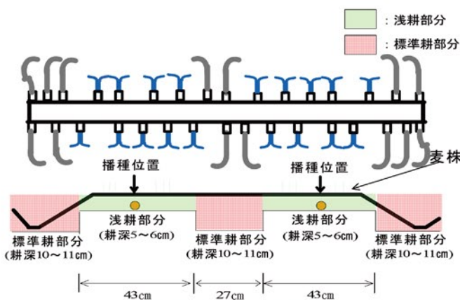
図1.ロータリ爪の配置例
