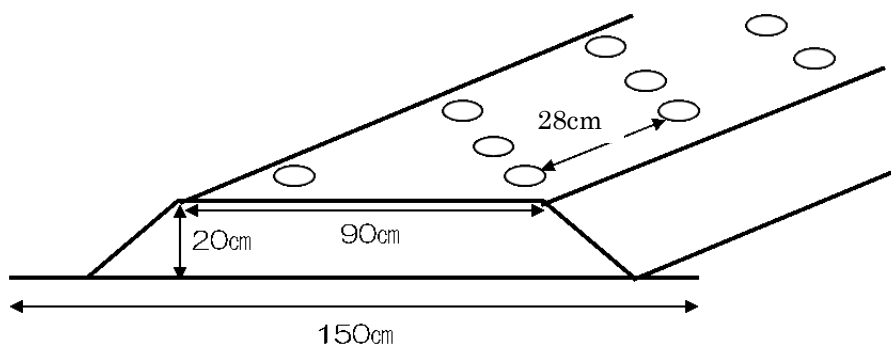
図3 畝立て図
